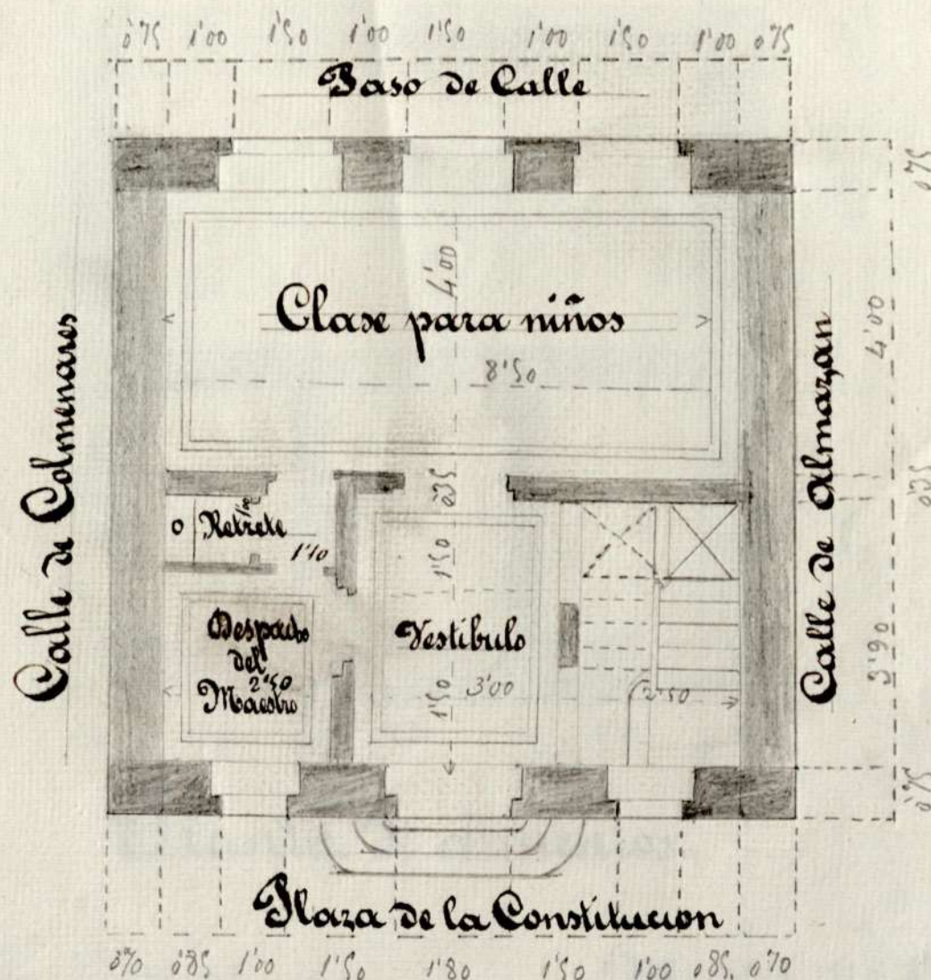
Planta baja.
